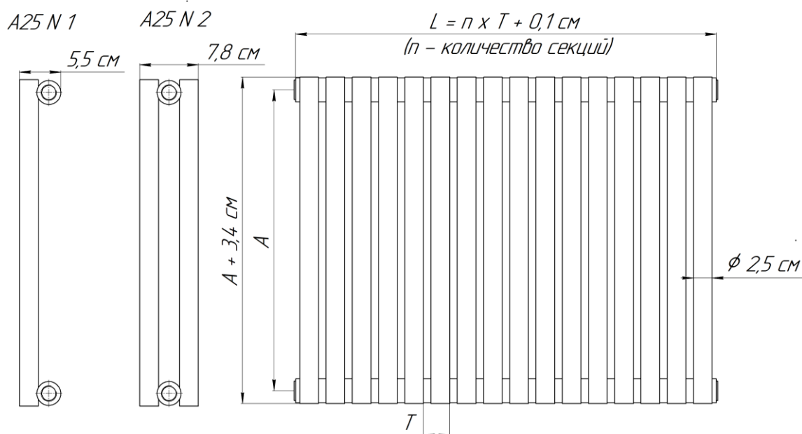
Рис 1. Радиатор «Гармония A25N», где: А – межцентровый размер, см; Т – шаг (Т = 3,5 см); n – количество секций; L – габаритная длина, см.
